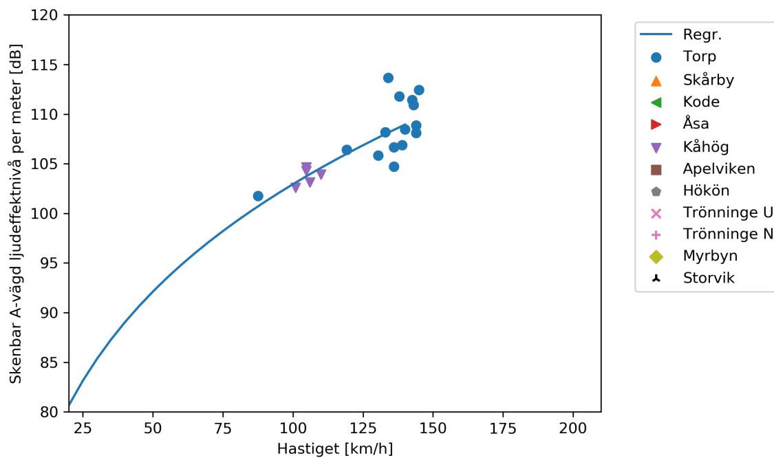
Figur 14: Beräknad och uppmätt skenbar A-vägd ljudeffektnivå per meter.
