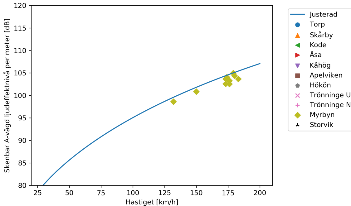
Figur 13: Beräknad och uppmätt skenbar A-vägd ljudeffektnivå per meter.
