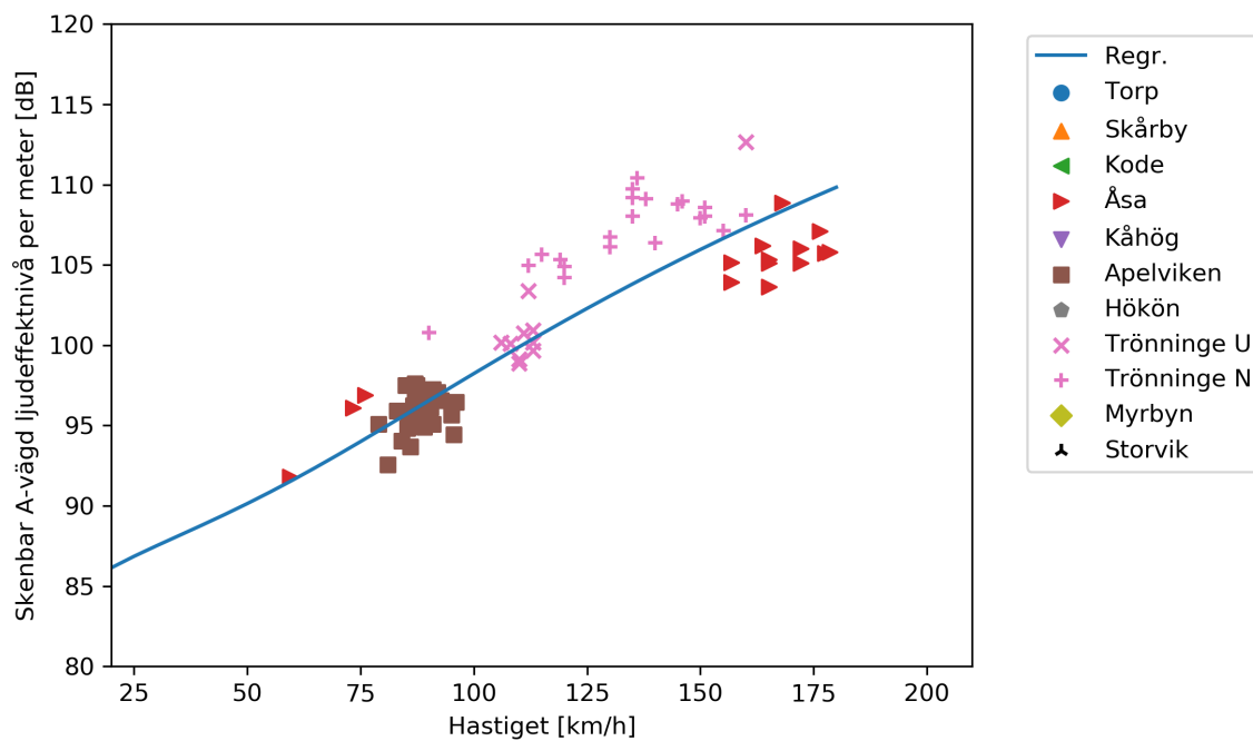
Figur 8: Beräknad och uppmätt skenbar A-vägd ljudeffektnivå per meter.
